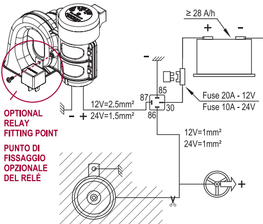
WIRING DIAGRAM WITH "HOT" LEAD TO HORN BUTTON SCHEMA DI MONTAGGIO CON BOTTONE DI COMANDO AL POSITIVO
