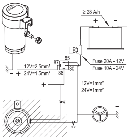
WIRING DIAGRAM WITH GROUND LEAD TO HORN BUTTON SCHEMA DI MONTAGGIO CON BOTTONE DI COMANDO A MASSA
