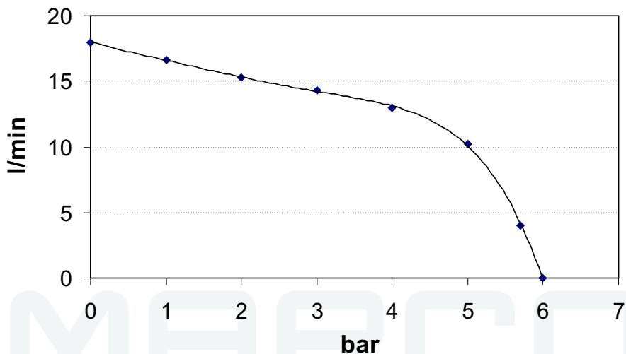
DIAGRAMME DE DÉBIT FLOW RATES DIAGRAM
