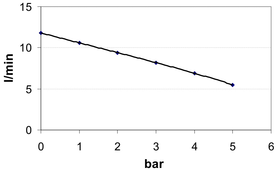
DIAGRAMME DE DÉBIT FLOW RATE DIAGRAM
